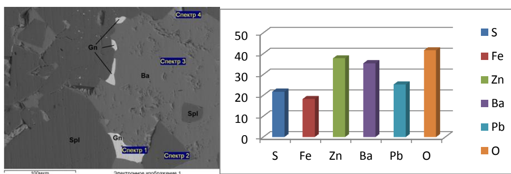
Рисунок 3 - Электронно-микроскопическое изображение состава руд в отраженном свете. % содержание компонентов в аншлифе: Gn - галенит; Ba - барит; Spl – сфалерит
