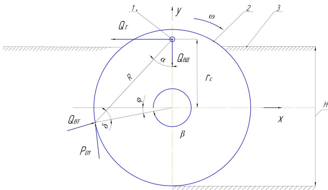
Сурет – Күштер сұлбасы: 1 – фрезаны ілу нүктесі; 2 – кесуші фреза; 3 – топырақ
