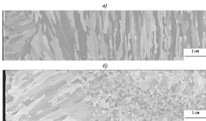
Рисунок 3 - Макроструктура продольного среза образцов экспериментального сплава, обработанных по методике «голубого» травления: а – слиток 1 (донная часть); б – слиток 3 (верхняя часть)
