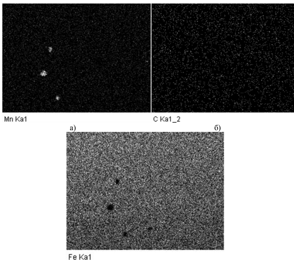
Рисунок 4 – РЭМ-изображения образца № 3 стали 20ГЛ после облучения электрическим импульсом и элементное картирование: а – Mn; б – С; в - Fe
