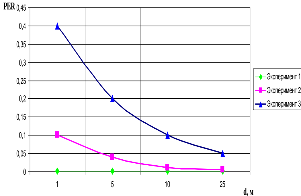
Рисунок 5 – Коэффициент ошибок пакетов PER в сети IEEE 802.15.4/ZigBee при шумовом воздействии сети IEEE 802.11 (Wi-Fi)
