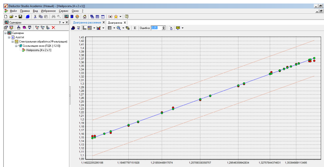
Рисунок 4 - Диаграмма рассеяния
