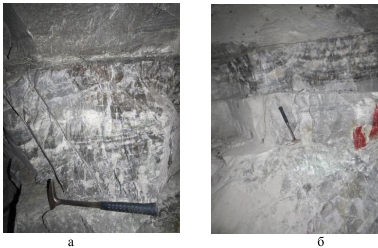
Рисунок 2 – Породы маслянской свиты: а - кремнистые алевролиты верхней пачки маслянской свиты на контакте с телом диабазовых порфиров; б - контакт алевролитов и кварцитов
