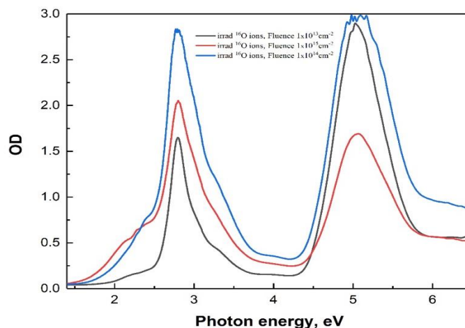
Рисунок.2 Спектры ОП LiF, облученного ионами кислорода ^{16}O с энергией 28 МэВ, измеренные при комнатной температуре после облучения
