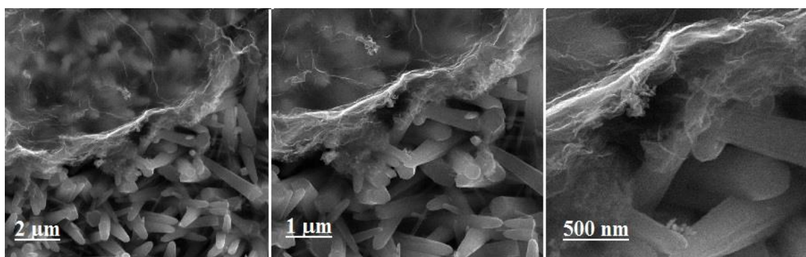
Рисунок 2. СЭМ изображения нанокompозита TNR/rGO
