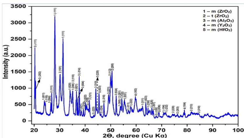
Сурет 3. 6YSZ – \text{Al}_2\text{O}_3 – \text{HfO}_2 бастапқы ұнтағының рентгенофазалық талдау нәтижесі
