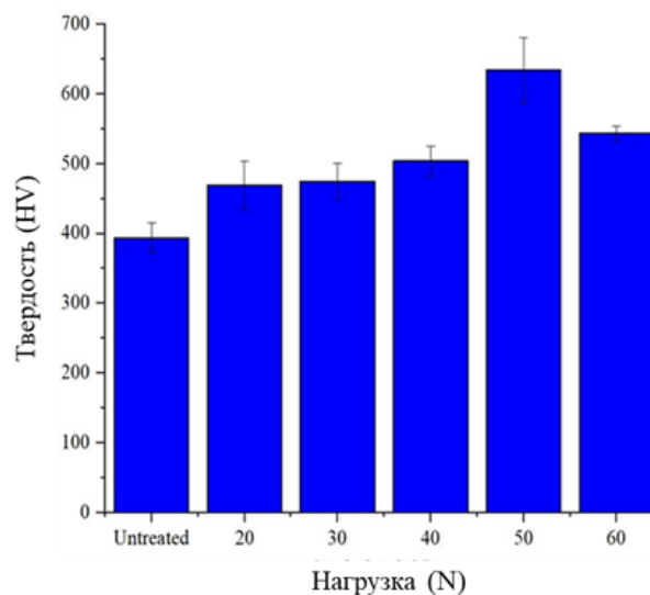
Рисунок 4. Изменение твердости образцов из сплава Ti6-Al-4V при пяти различных нагрузках (20, 30, 40, 50, 60 Н)
