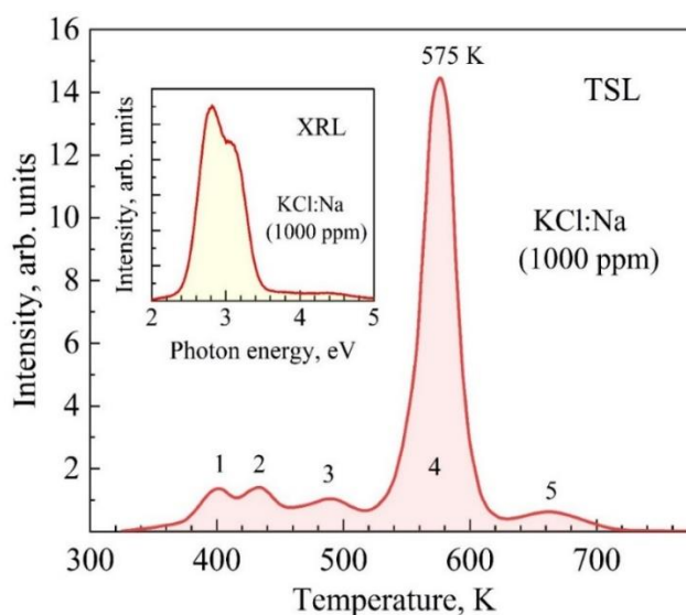
Рисунок 3. ТСЛ и спектр РЛ (на вставке) изодозно облученных закаленного KCl:Na
