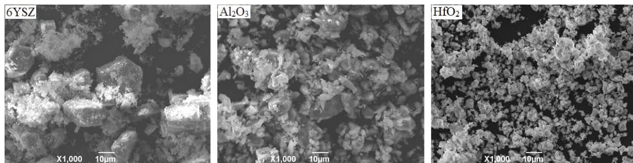
Сурет 1. 6YSZ, Al_2O_3 және HfO_2 ұнтақтарының СЭМ-кескіні
