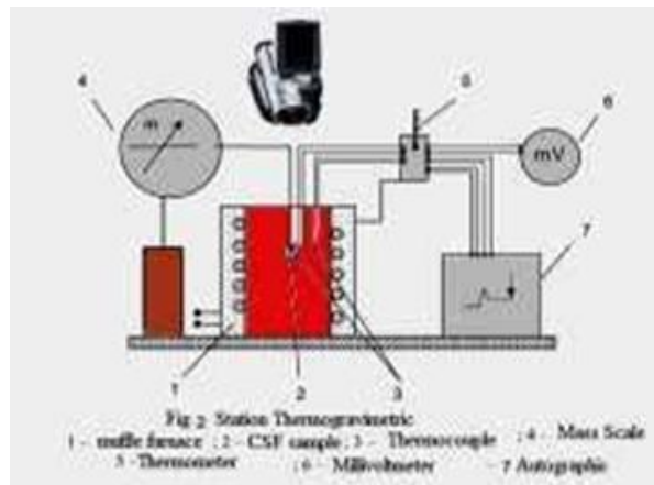
Рисунок 3. Термическое поведение различных составов композитного топлива изучается на термогравиметрической станции при нормальном атмосферном давлении для определения подходящего состава композитного топлива
