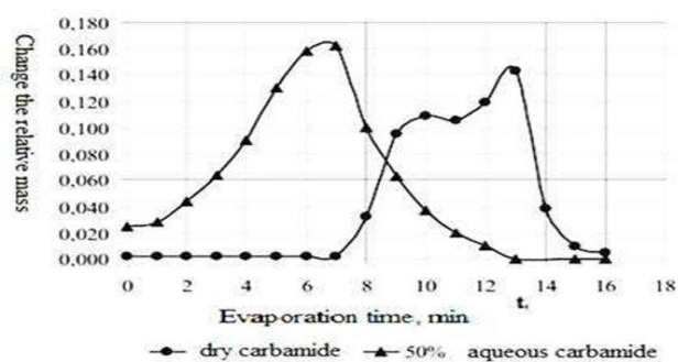
Рисунок 6. Изменение относительной массы действующего вещества в зависимости от испарения время как в твердом состоянии, так и в водном растворе
