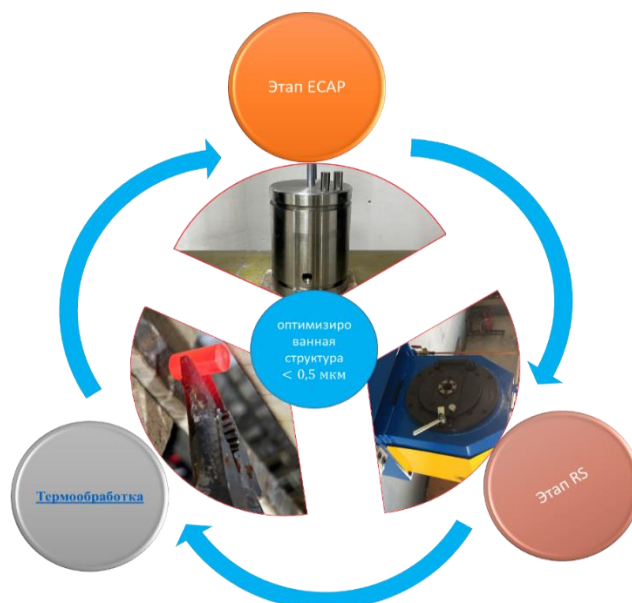
Рисунок 4. Схема этапов комбинированной обработки ЕСАР и RS с промежуточной термической обработкой
