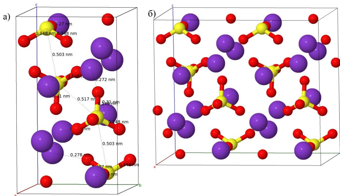
Рисунок 1. Структура элементарной ячейки (а) и суперячейки (б) \beta\text{-K}_2\text{SO}_4
