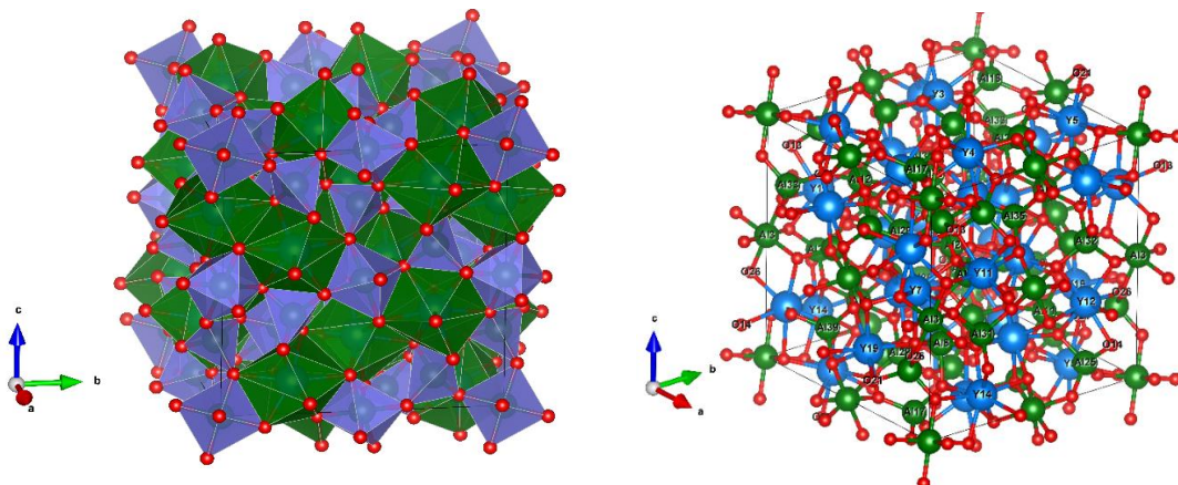
1-сурет. Полиэдрлік құрылымындағы иттрий-алюминий-гранатының кристалдық құрылымы. Сурет Vesta бағдарламасында жасалынды
