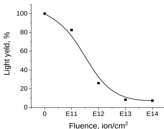
Рисунок 5. Световыход фотолюминесценции кристаллов \text{CaF}_2:\text{Eu} облученных ионами 220 МэВ ^{132}\text{Xe} до флюенсов от 10^{11} до 10^{14} ион/см 2 , при 300 К
