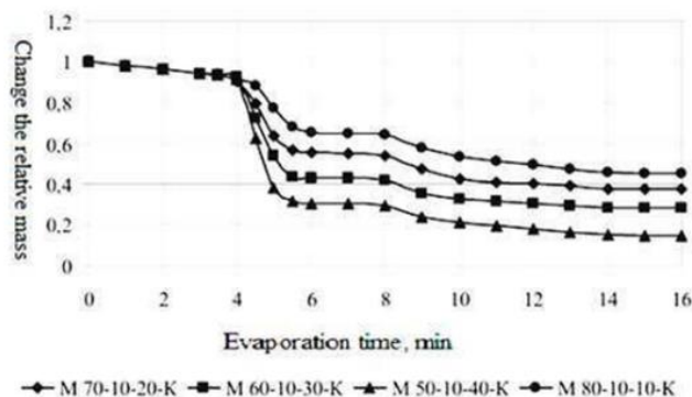
Рисунок 8. Влияние добавления карбамида в ВУТ
