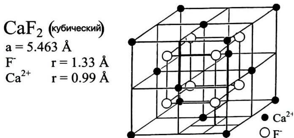
Рисунок 1. Структура кристаллов \text{CaF}_2 . Параметры кристаллической решетки
