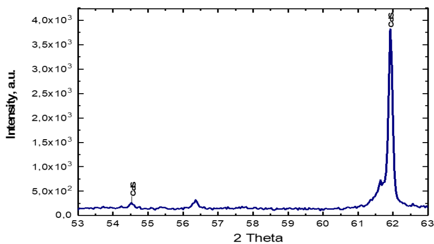
Сурет 2. CdS наносым үлгілерінің рентгенографиясы: тұндыру уақыты 30 мин, T=70° C
