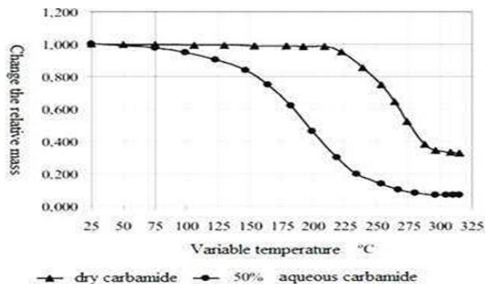
Рисунок 7. Изменение относительной массы карбамида при постепенном повышении температура
