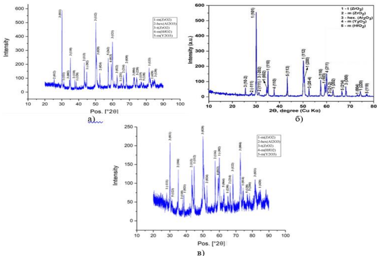
Сурет 4. Күйдірілген үлгінің рентгенофазалық талдау нәтижелері: а) T = 1400^{\circ}\text{C} , б) T = 1500^{\circ}\text{C} , в) T = 1600^{\circ}\text{C}
