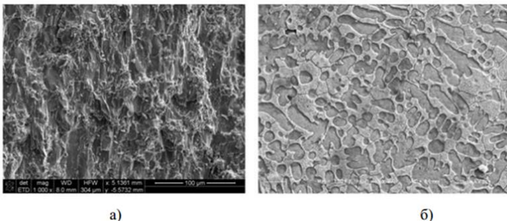
Сурет 2. Қорытпа құймалары бетінің СЭМ көмегімен алынған суреттері: а) \text{CrNbVTiZr} б) \text{FeCoCuNiSn}_{0.5} [15]
