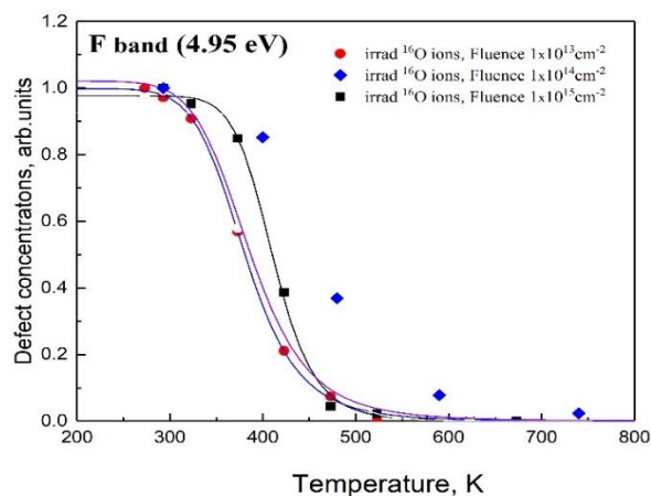
Рисунок 4. Зависимость оптического поглощения в разных спектральных областях от температуры промежуточных прогрева для кристалла LiF облученных ионами кислорода 16 O
