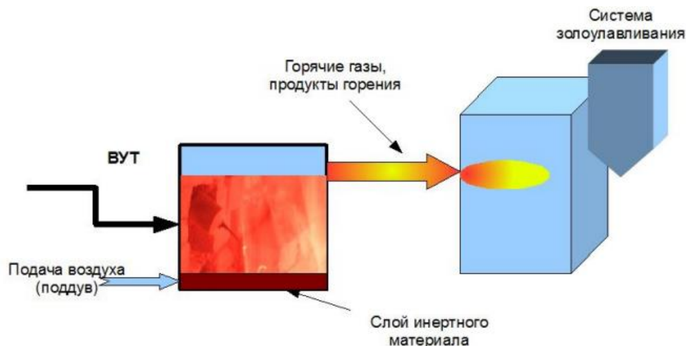
1-сурет. СКО-ң қайнаған қабатта жағу
