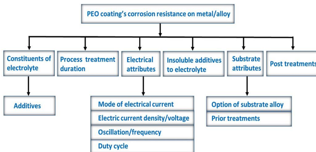
Рисунок 4. Условия обработки в коррозионной сопротивлении покрытий РЕО. Адаптировано из [41].
