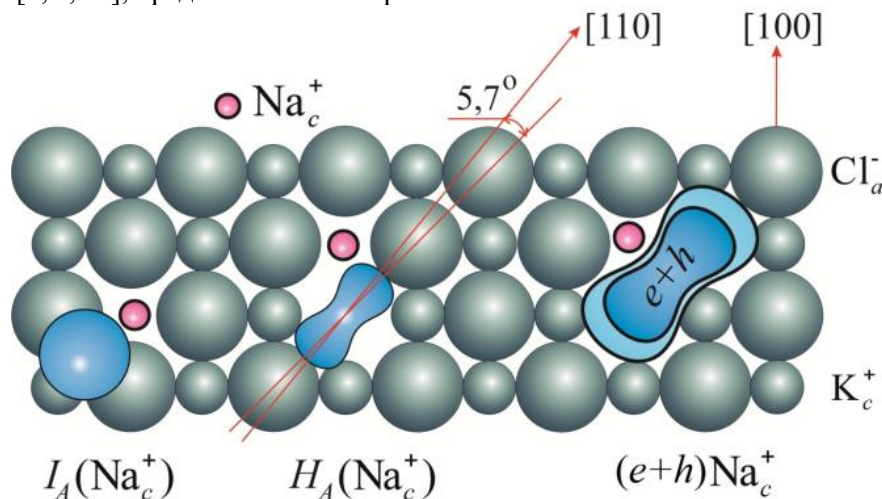
Рисунок 5. Модели I_A(\text{Na}_c^+) -, H_A(\text{Na}_c^+) -центров и (e+h)\text{Na}_c^+ около примесного иона в KCl:Na.
