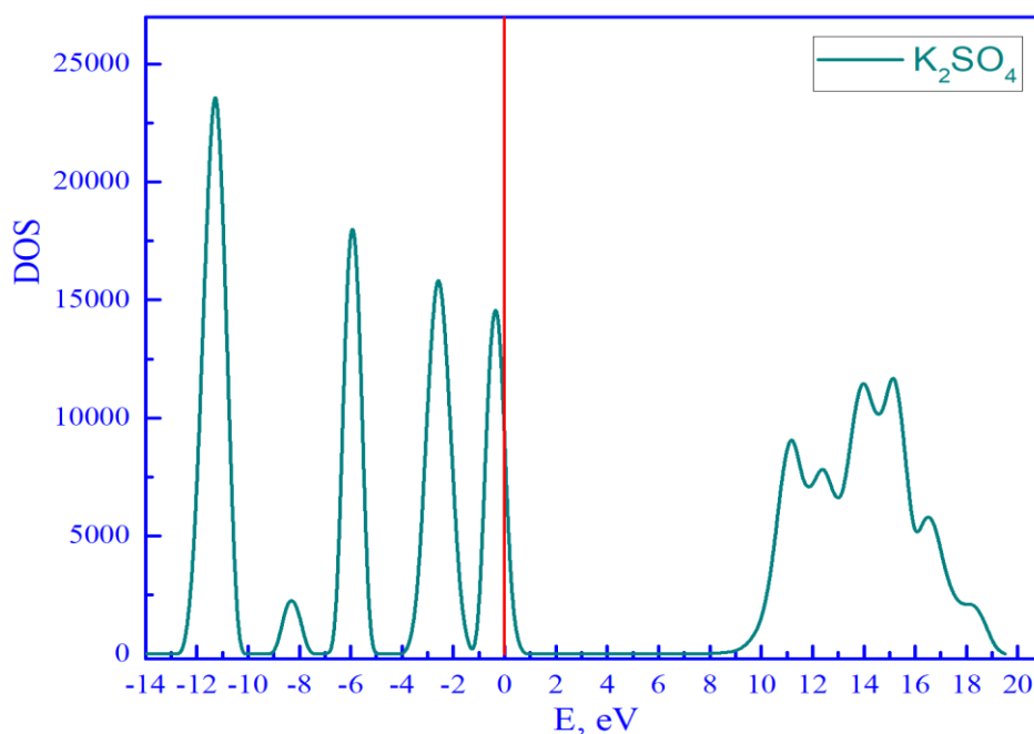
Рисунок 2. Плотность электронных состояний \beta\text{-K}_2\text{SO}_4
