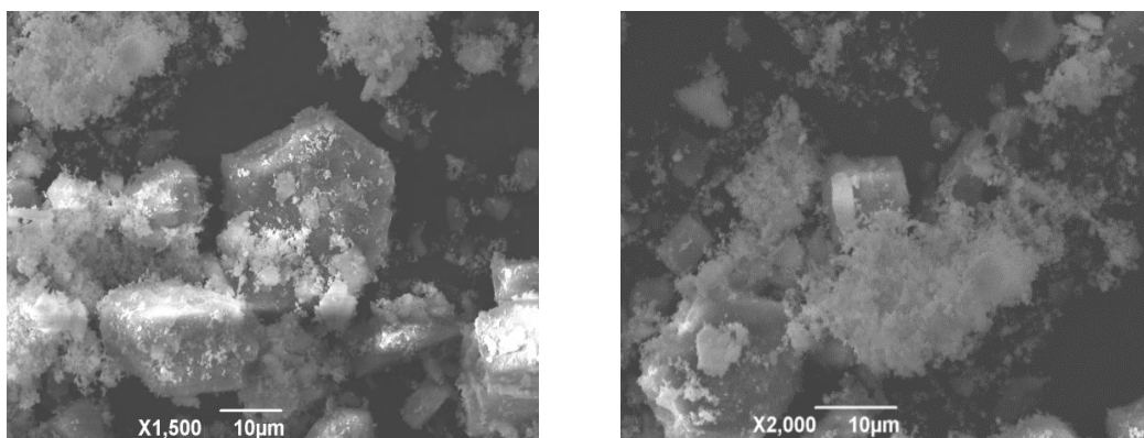
Сурет 2. 6YSZ – \text{Al}_2\text{O}_3 – \text{HfO}_2 ұнтақ қоспасы бөлшектерінің электрондық кескіні
