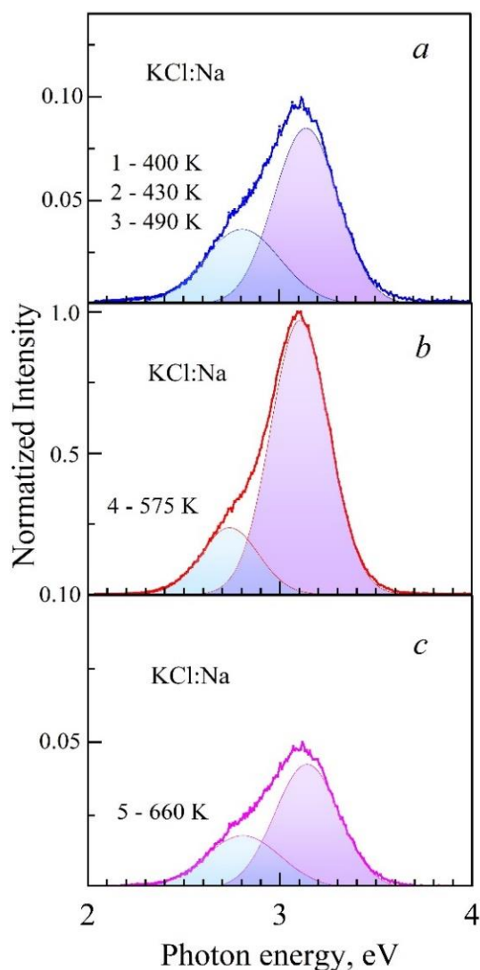
Рисунок 4. Спектры ТСЛ закаленного \text{KCl}:\text{Na} , зарегистрированные в пиках, указанных на рис. 3: а – при 400 К (1), 430 К (2), 490 К (3); б – при 575 К (4); с – при 660 К (5)
