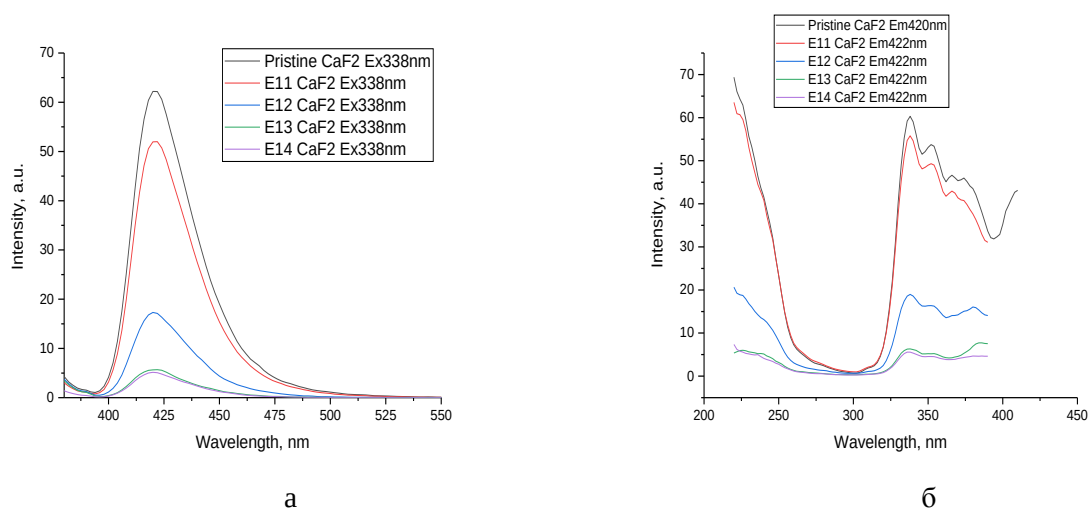
Рисунок 4. Спектры фотолуминесценции (а); спектры возбуждения (б) кристаллов \text{CaF}_2 : Eu облученных ионами 220 МэВ ^{132}\text{Xe} до флюенсов от 10^{11} до 10^{14} ион/см ^2 , при 300 К
