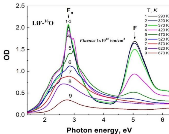
Рисунок.3 Спектр оптического поглощения кристалла LiF облученного ионами кислорода 16 O с энергией 28 МэВ с флюенсами от \Phi=1 \times 10^{13} ион/см 2 до \Phi=1 \times 10^{15} ион/см 2 после ступенчатого нагрева от 293 К до 750 К
