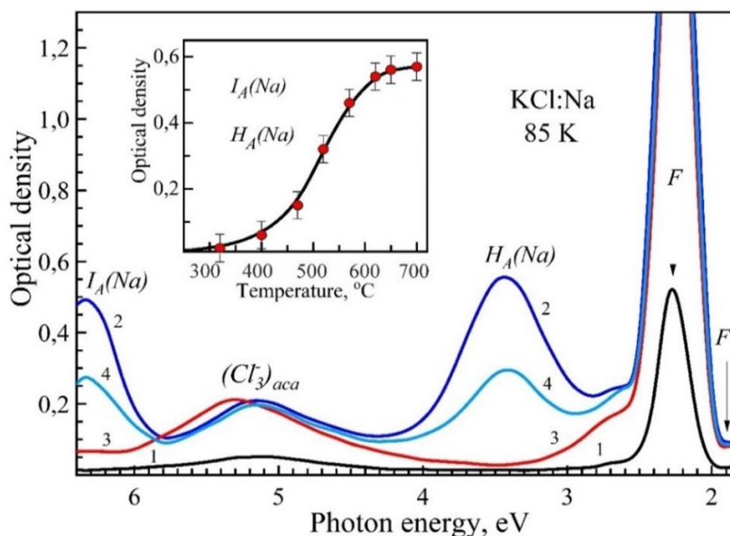
Рисунок 1. Спектры поглощения при 85 К радиационных дефектов в изодозно облученных (3 ч, 20 мА, 45 кВ, W-антикатод) кристаллах: 1 – KCl; 2 – свежесращенного KCl:Na, 3 – KCl:Na, хранившегося более 3-4 месяца при комнатной температуре, 4 – KCl:Na после закалки до 600°C с выдержкой 15 минут. На вставке представлена зависимость спектров поглощения I_A(\text{Na}_c^+) - и H_A(\text{Na}_c^+) -центров в кристаллах KCl:Na от температуры закалки
