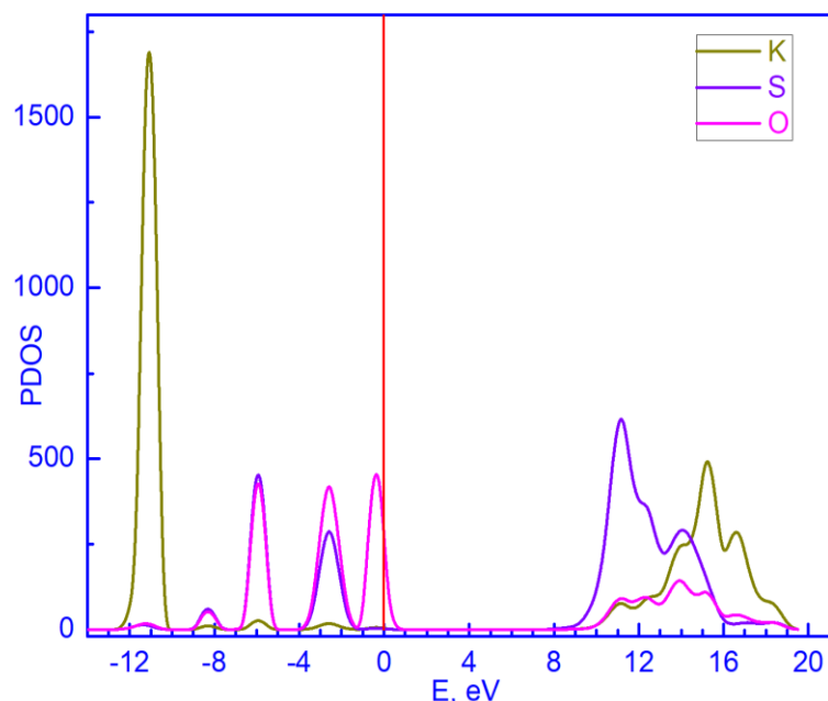
Рисунок 3. Парциальная плотность электронных состояний \beta -K 2 SO 4
