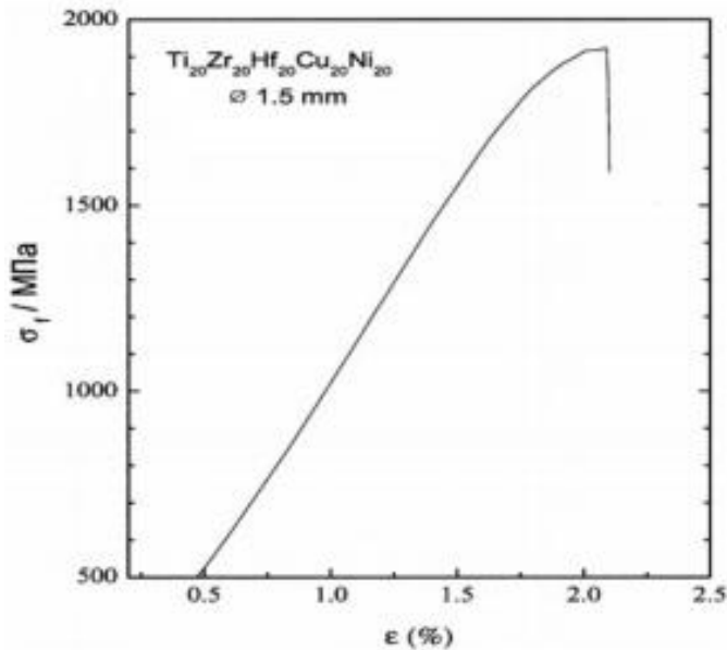
Сурет 5. TiZrHfCuNi аморфты қорытпасының сығылу кезіндегі кернеу мен деформация қисықтары [20]
