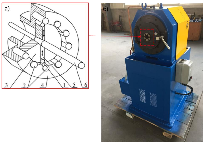
1,2 — ролики; 3 — штибель; 4 — обойма; 5 — бойки; 6 — заготовка Рисунок 3. Схема ротационнойковки (а) и ротационно-ковочная машина (б)
