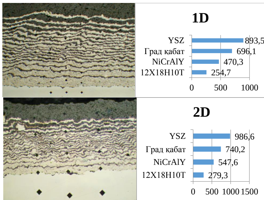
4-сурет. NiCrAlY/ZrO 2 -Y 2 O 3 градиентті жабындарының көлденең қимасы және микроинденттеу іздері: а) 1D режимі, б) 2D режимі
