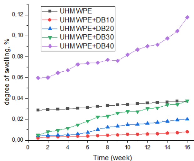
Рисунок 2. Временные зависимости стабильности покрытия композитные покрытия СВМПЭ с разным процентным содержанием диабаз в 10 мас% соляной кислоте
