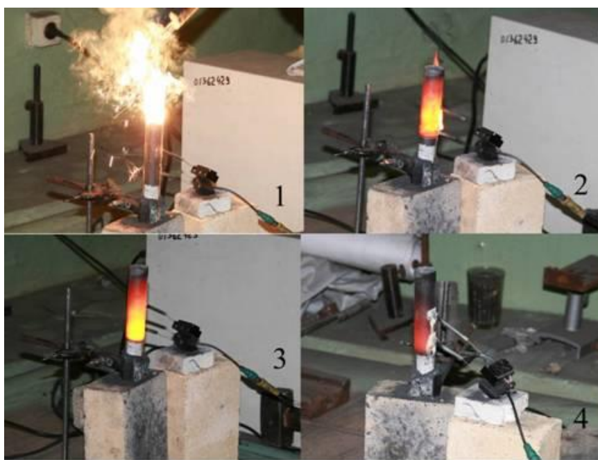
Рисунок 2. Последовательность прохождения СВС. 1 - пожег смеси. 2 - горение смеси. 3 - остановка движения фронта горения. 4 - остывание смеси
