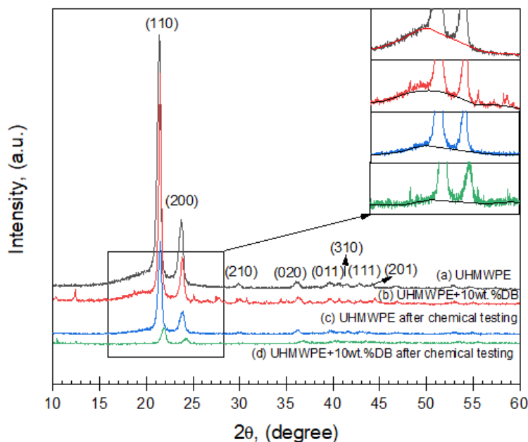
Рисунок 4. Рентгеновские дифрактограммы образцов из чистого СВМПЭ и композита СВМПЭ с диабаз наполнителем с содержанием 10 мас.% в исходном состоянии и после воздействия кислотной среды
