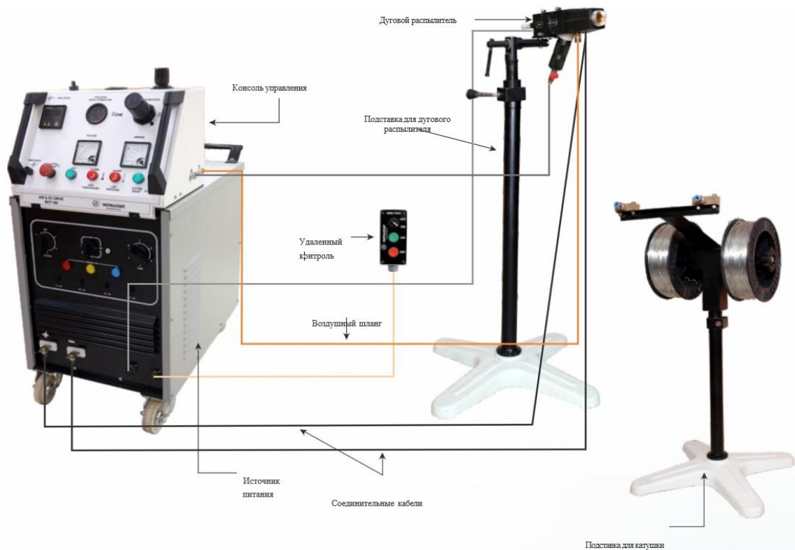
Рисунок 1. Схема системы дугового распыления
