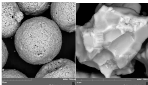
1-сурет. YSZ (а) және NiCrAlY (b) ұнтақтарының морфологиясы
