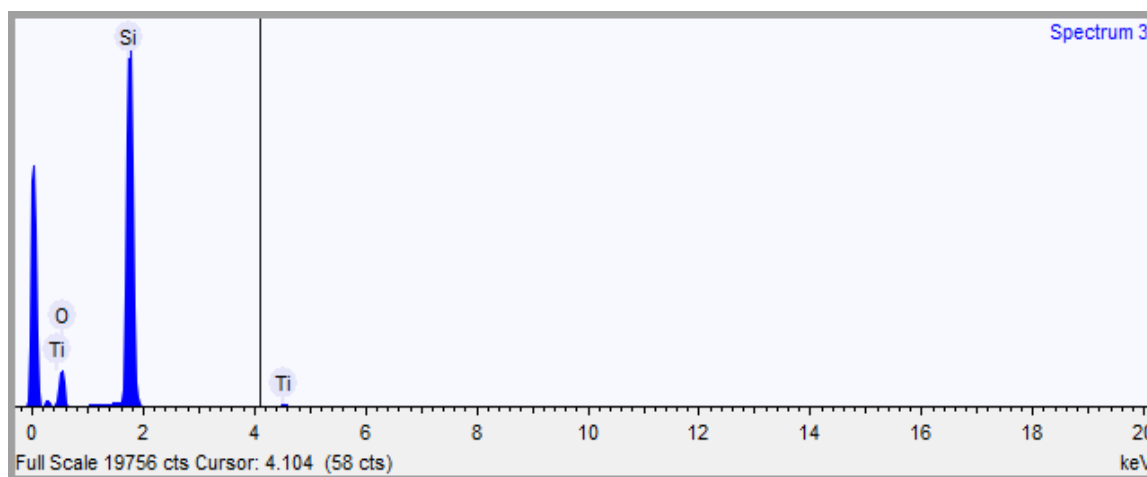
Сурет 2. Синтезделген үлгілерді EDX талдау
