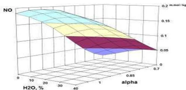
Рисунок 10. Содержание NO в продуктах сгорания, измеренное при использовании различных топливных смесей с переменными по сравнению с Альфа
