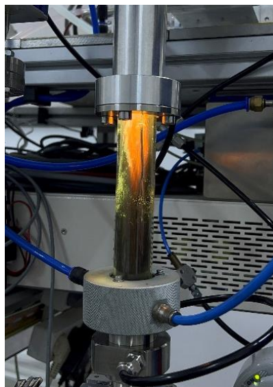
Рисунок 1. Реакционная камера во время эксперимента
