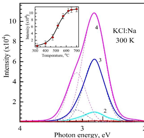
Рисунок 2. Спектры РЛ \text{KCl}:\text{Na} (100 ppm), измеренные при комнатной температуре до (кривая 1) и после закалки при 400°C (кривая 2), 520°C (кривая 3) и 700°C (кривая 4). На вставке представлена зависимость интенсивности полосы люминесценции с максимумом при 2,8 эВ от температуры закалки кристалла
