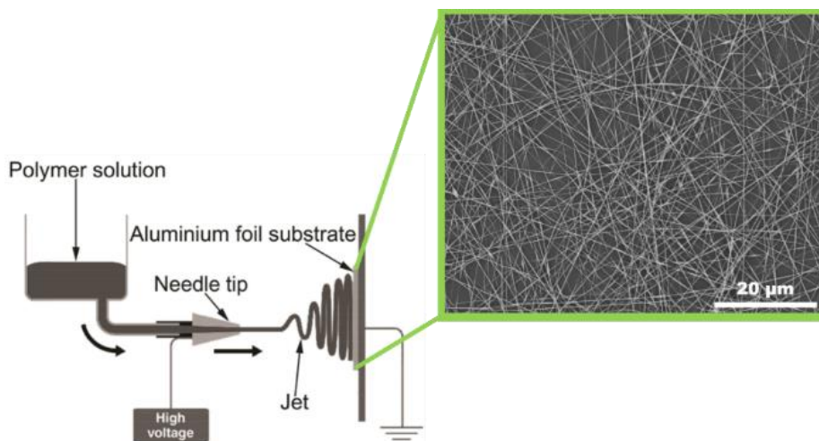
Сурет 3. Электроспиннинг әдісімен наноталшық алу диаграммасы
