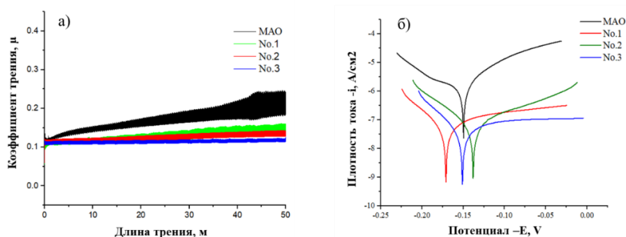
Рисунок 3. Трибологические и электрохимические свойства покрытий, полученных методом микродугового оксидирования
