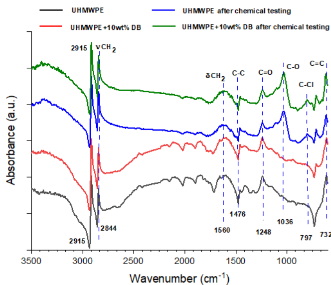
Рисунок 3. ИК-спектры образцов из чистого СВМПЭ и с 10 процентным диабаз-наполнителем до и после воздействия кислотной среды
