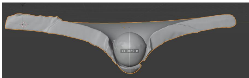
Рисунок 2. Цифровая модель контактного взаимодействия шара и медной пластины
