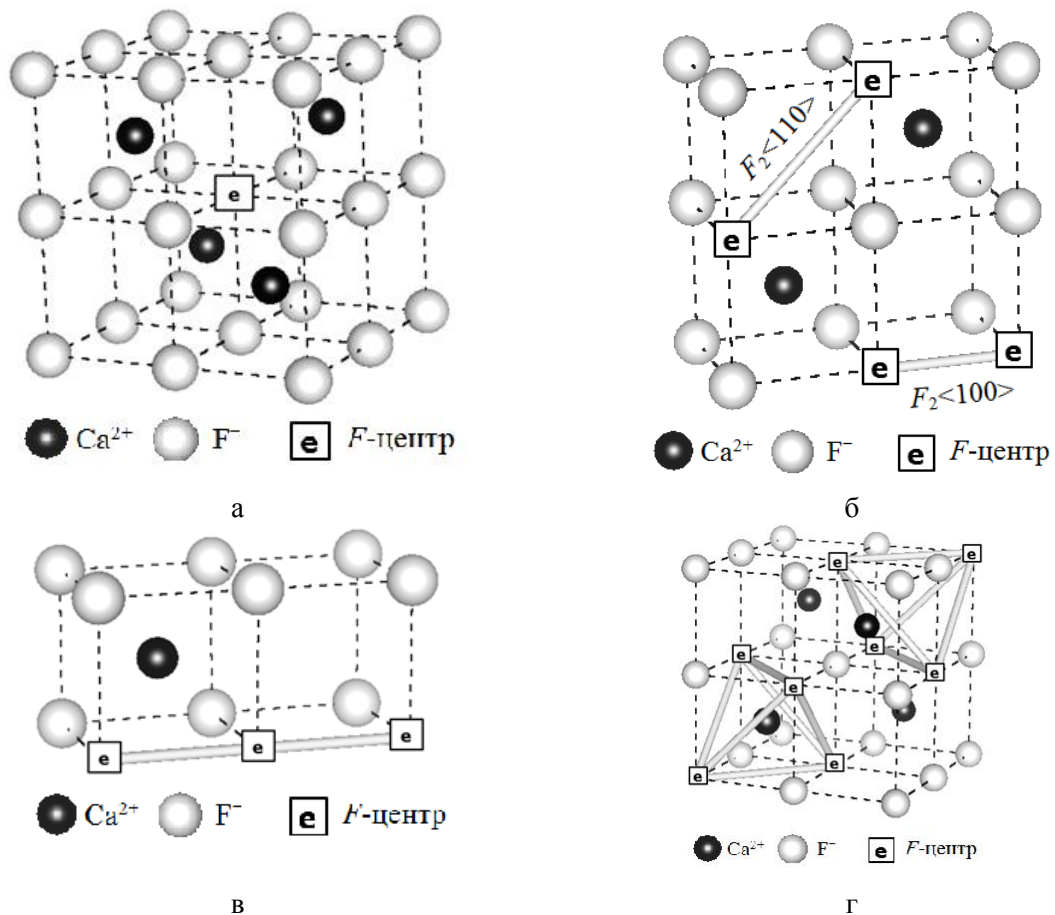
Рисунок 3. Схематическое изображение основных электронных центров окраски в кристаллах \text{CaF}_2 : а) F центр; б) F_2 центр; в) F_3 центр; г) F_4 -центр
