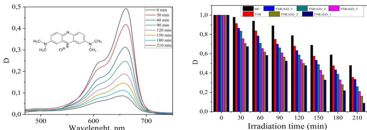
Рисунок 3. Деградация красителя МС в присутствии образцов TNR и TNR/rGO
