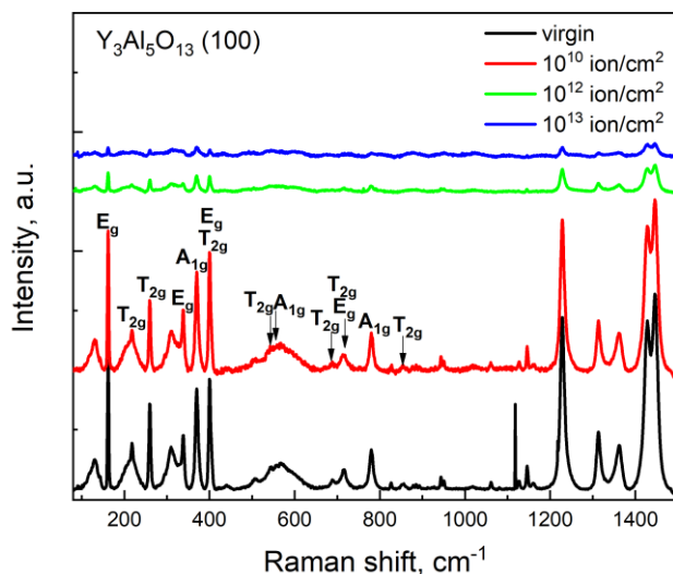
3-сурет. (100) бағытындағы YAG монокристалының Раман спектрлері, бөлме температурасында 230 МэВ энергиялы Хе иондарымен және флюенстері 10^0 – 10^{13} ион/см 2 дейінгі диапазонда сәулелендірілген
