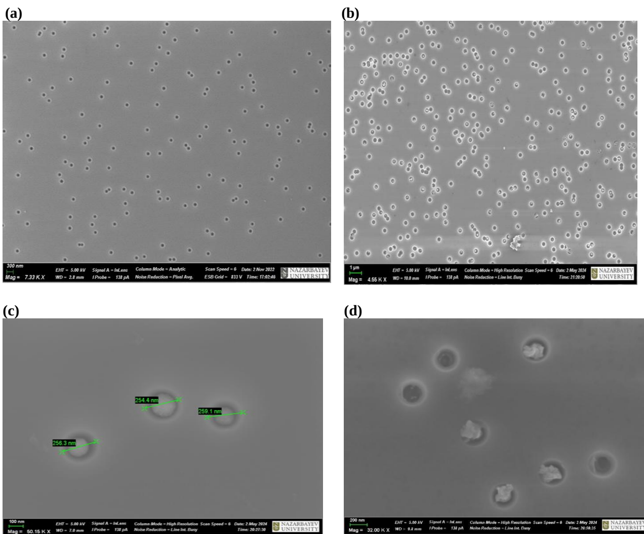
Сурет 1. SiO 2 /Si трек шаблондарында CdS наносымдарын СЭМ суреттері: (а) химиялық тұндыруға дейінгі, (b,c) және (d) химиялық тұндырудан кейінгі. Тұндыру уақыты 30 минут, T=70° C
