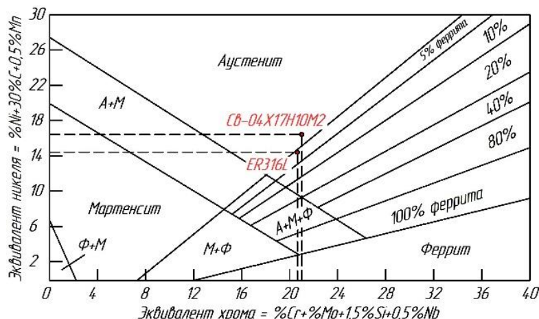
Рисунок 2. Содержание феррита в металле шва на диаграмме Шеффлера при сварке сталей 12Х18Н10Т с AISI 316 для присадочной проволоки Св-04Х17Н10М2 и ER316L
