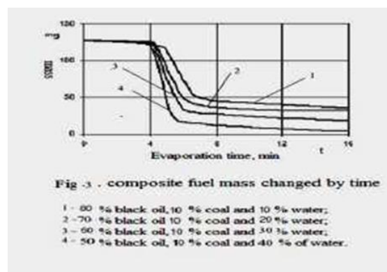
Рисунок 4. Результаты изменения массы композитного топлива во времени
