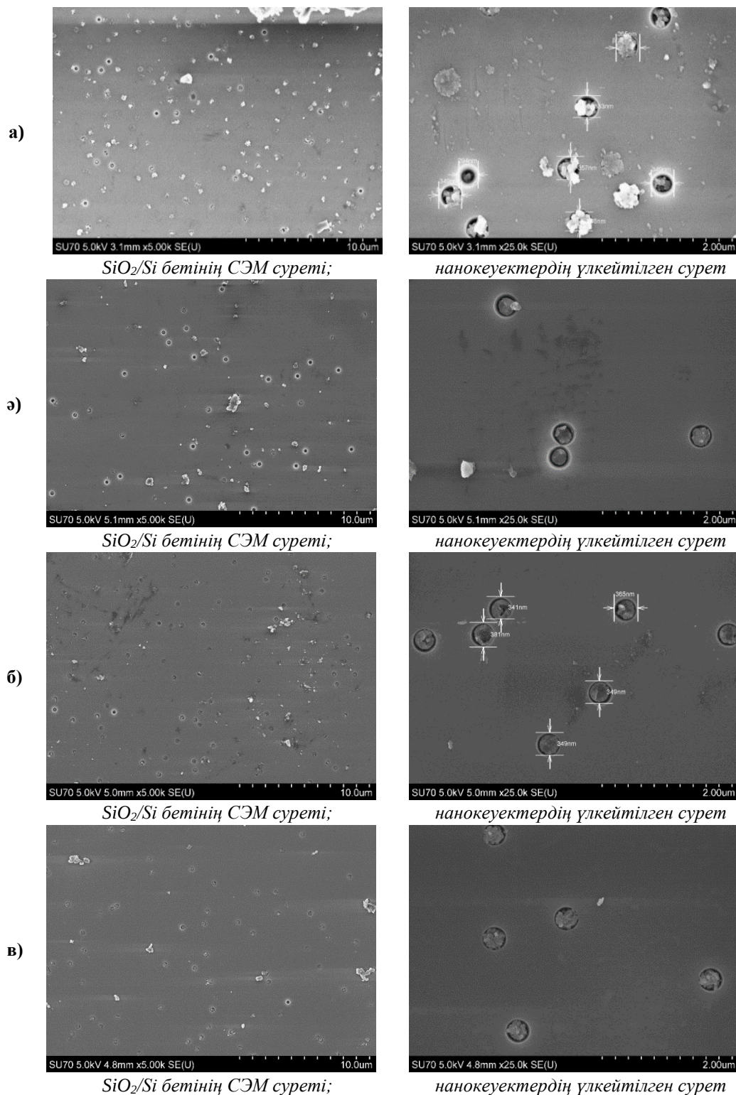
Сурет 1. Әртүрлі температурадағы золь-гель синтезінен кейінгі темплэйт бетінің СЭМ суреттері: а) 1 үлгі – 500 °С; ә) 2 үлгі – 600 °С; б) 3 үлгі – 700 °С; в) 4 үлгі – 800 °С
