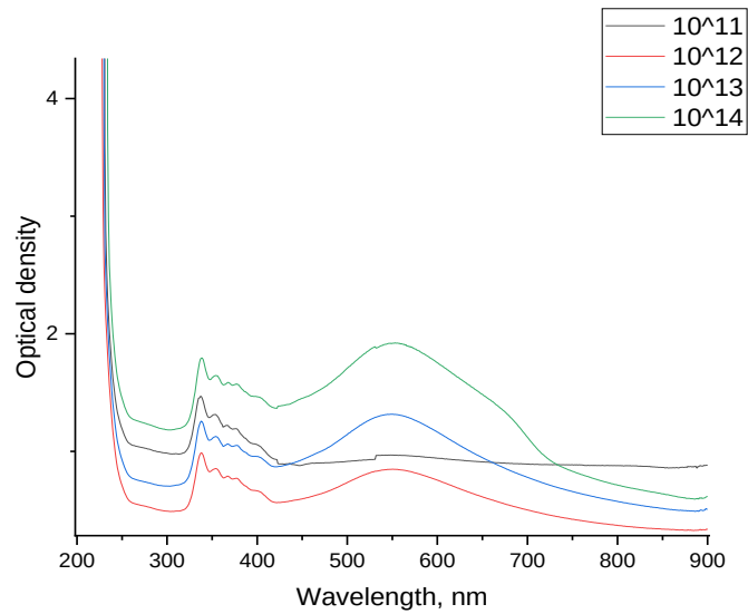
Рисунок 2. Спектры поглощения кристаллов \text{CaF}_2 : Eu облученных ионами 220 МэВ ^{132}\text{Xe} до флюенсов от 10^{11} до 10^{14} ион/см ^2 , при 300 К
