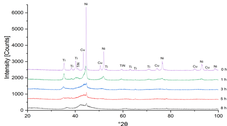
Рисунок 1. Дифрактограмма порошков NiTi45Cu10 после механосинтеза при 750 об/мин
