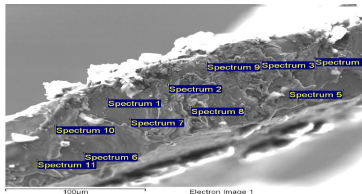
Рисунок 4. Точки энергодисперсионного анализа по толщине пленки
