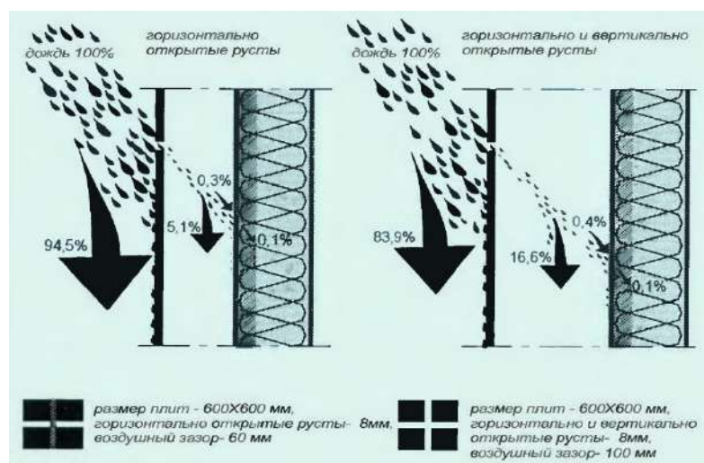
Рисунок 2. Схема воздействия ливневого дождя на фасад
