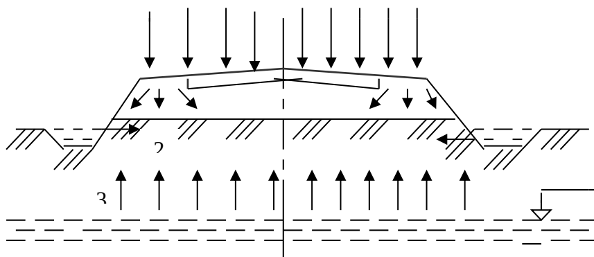
Рисунок 1. Основные источники увлажнения дорожной
