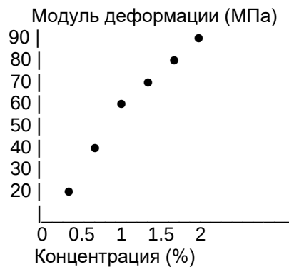
Рисунок 2. Модуль деформации
