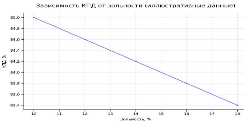
Рисунок 1. Зависимость КПД от зольности угля
