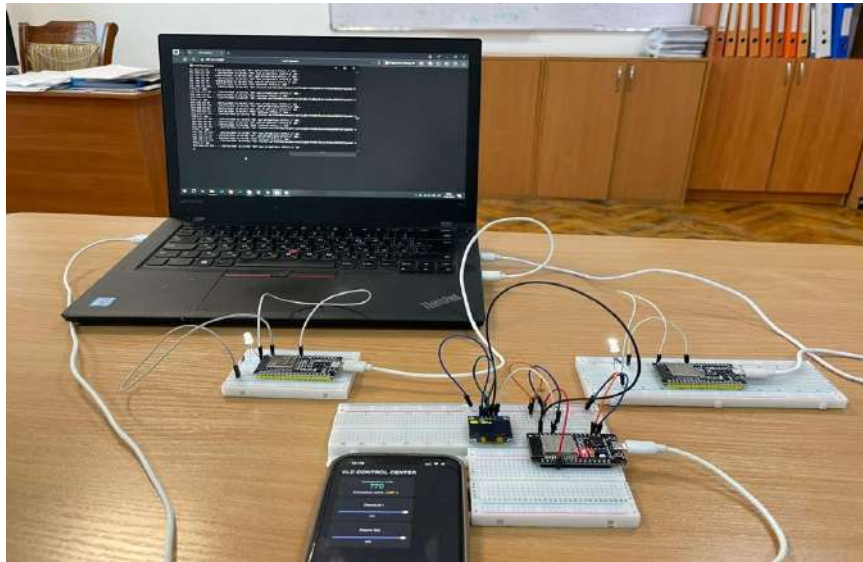
Рисунок 4. Экспериментальный стенд
