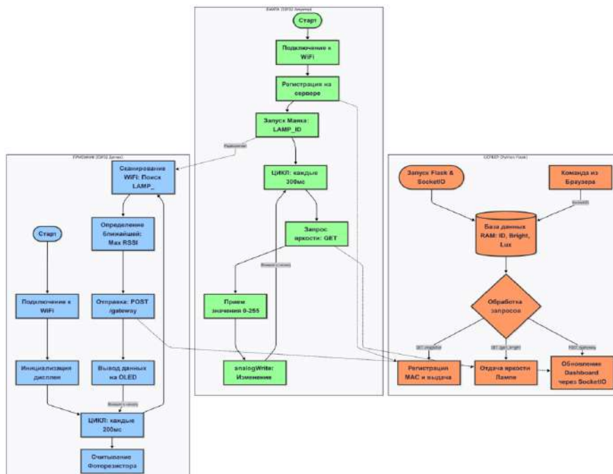
Рисунок 3. Алгоритм работы системы
