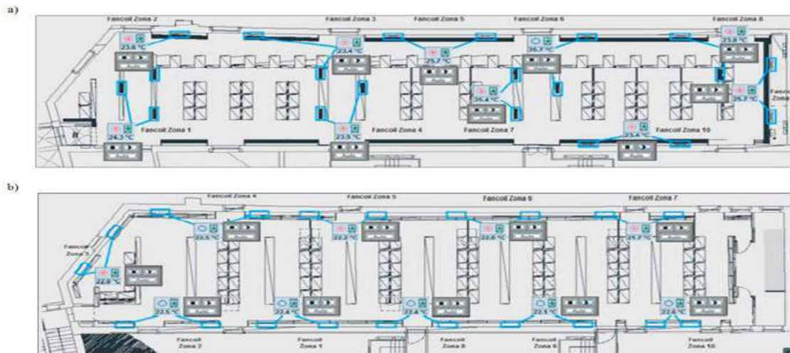
Рисунок 3.1. Размещение фанкойлов (а) комната «С», (б) комната «Д» [5]
