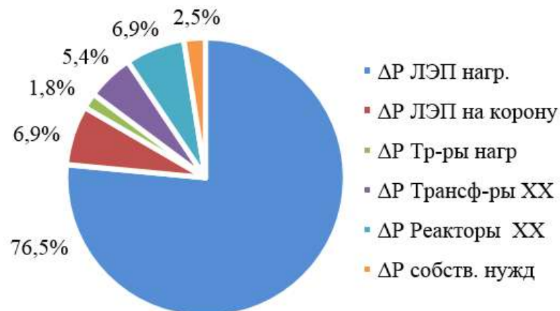
Рисунок 2. Диаграмма структуры технических потерь электрической мощности Восточного энергорегиона РК
