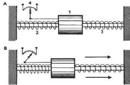
Сурет 1. Акселерометрдің жұмыс істеу механизмі
