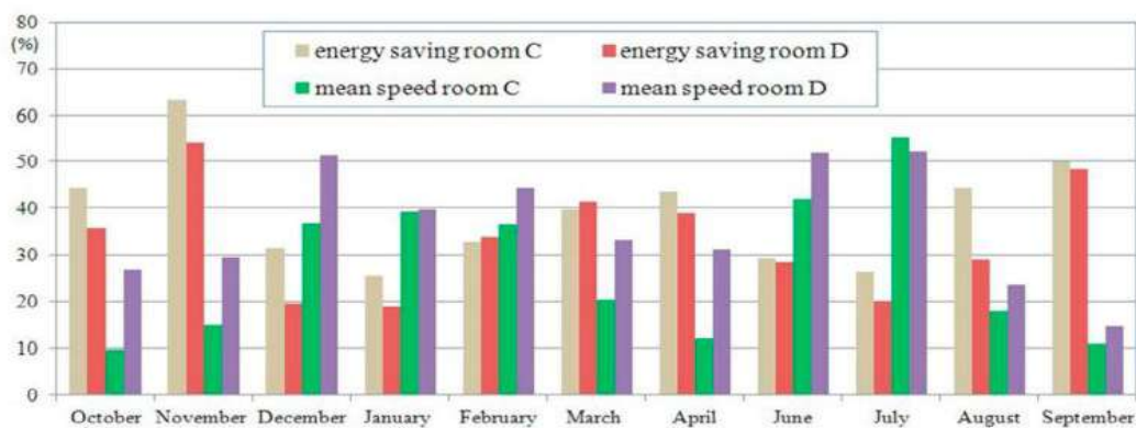
Рисунок 3.2. Среднемесячные значения оборотов вентилятора в процентах от полной скорости в помещениях С и D соответственно и соответствующий процент экономии энергии за разные месяцы. [5]
