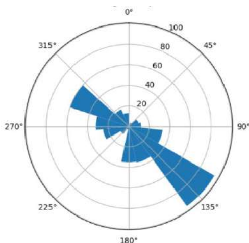
Рисунок 2. Роза ветров по месяцам
