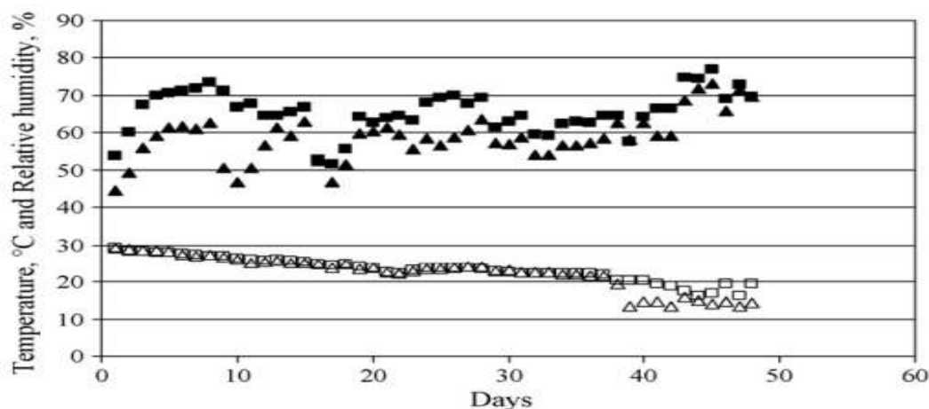
Рисунок 2.2 График температуры и влажности в помещениях при применении VSD (Δ, ▲) и при прямом пуске (□, ■) [4]
