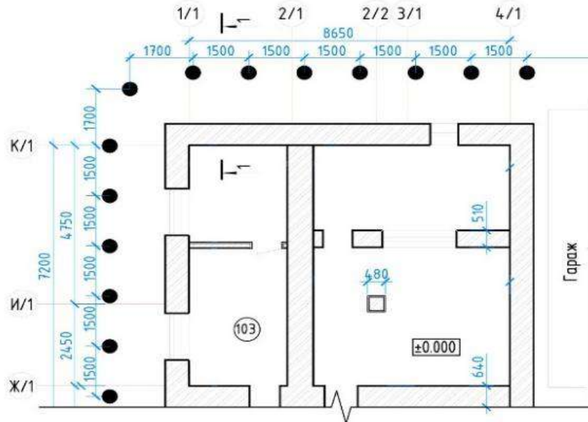
Рисунок 2. Схема расположения скважин в осях Ж/1 – К/1 и 1/1 – 4/1
