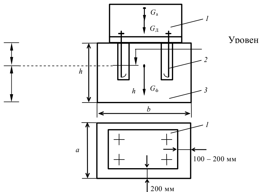
1 – аппарат; 2 – фундаментный болт; 3 – фундамент
