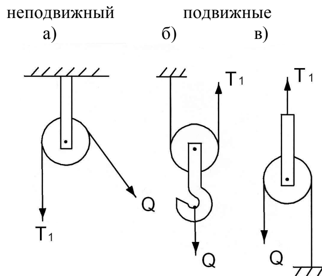
Рисунок 4 – Блоки
