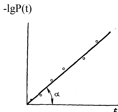
Рисунок 23 – Графический способ определения интенсивности отказов \lambda
