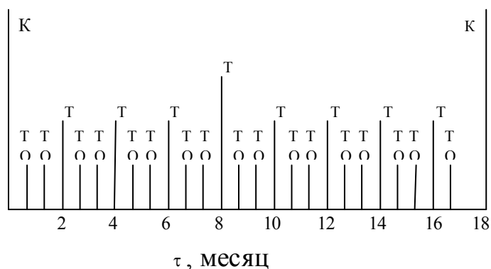
Рисунок 19 - Схема межремонтного цикла
