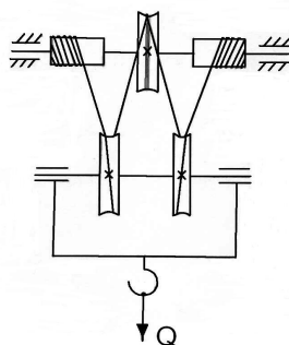
Рисунок 7 – Сдвоенный полиспаст
