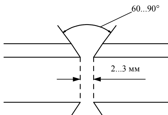
Рисунок 11 - Схема сварки труб
