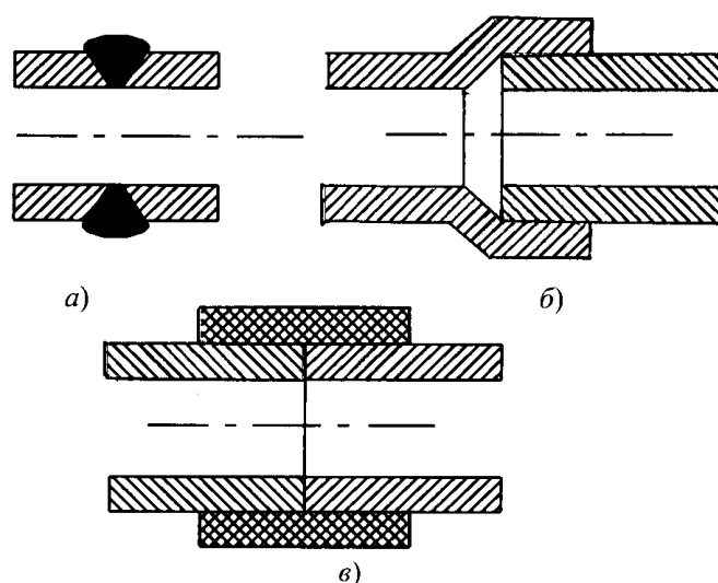
Рисунок 12 - Способы соединения труб
