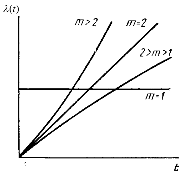
Рисунок 25 - Зависимость интенсивности отказов распределения Вейбулла
