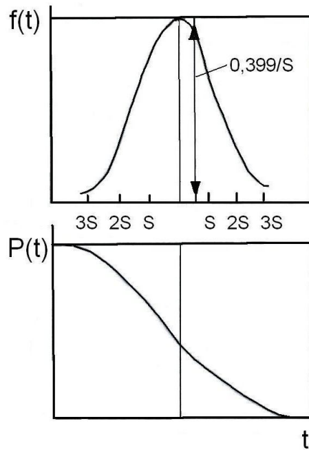
Рисунок 24 – График нормального распределения
