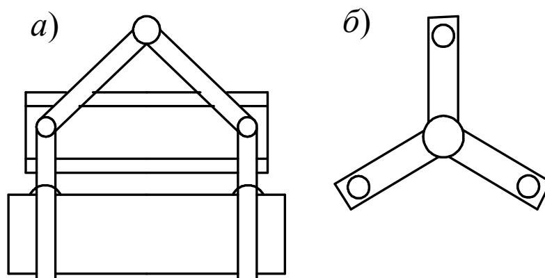
Рисунок 10 – Траверсы
