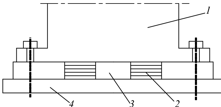
1 – оборудование; 2 – пакет пластин; 3 – подливка; 4 – фундамент Рисунок 3 - Установка оборудования на фундаменте
