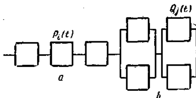
Рисунок 31 – Надёжность дублированной системы
