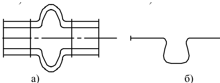
Рисунок 13 - Способы компенсации температурных напряжений
