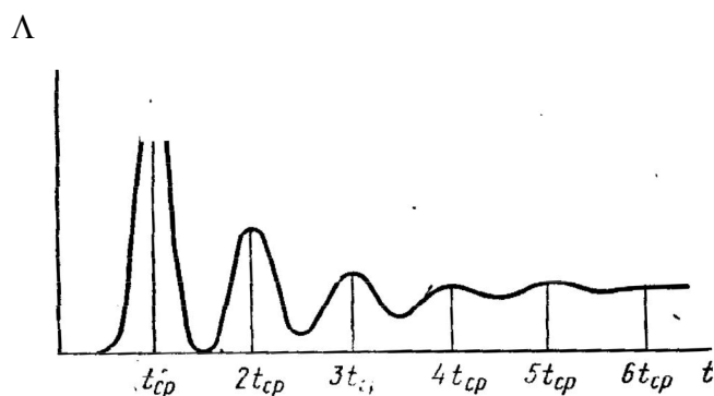
Рисунок 29 - График частоты отказов
