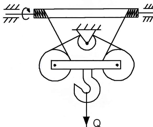
Рисунок 6 - Подвижный полиспаст
